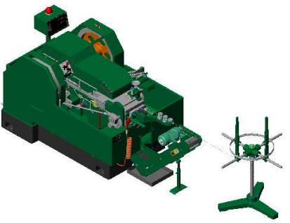
打頭機 H15-50-BH(高速)+檢測器+燈架
