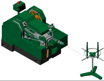
打頭機 H15-37-BH (高速)+檢測器+輸送機
