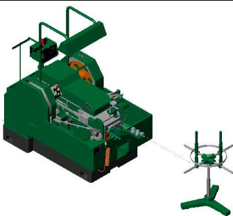
打頭機 H15-50-BH(高速)+檢測器+燈架+輸送機
